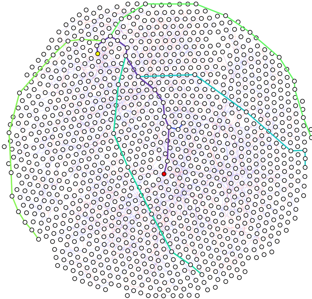
Figura D.3: Graf d'invariants j supersingulars per a p = 2^{13}3^7 - 1 = 17915903 . Per a aquest primer, hi ha 1492993 invariants supersingulars, dels quals només se'n mostren 1240. Les 2-isogènia estan representades de color vermell, i les 3-isogènia, de color blau. El node groc correspon a la corba E_0 amb j(E_0) = 1728 . El node vermell correspon a la clau pública d'Alice. L'escala de color de les isogènia ressaltades va del verd clar ( i = 1 ) al lila ( i = 13 ). Cada isogènia és la resultant de fer el quocient només coneixent els primers i bits de la clau.
